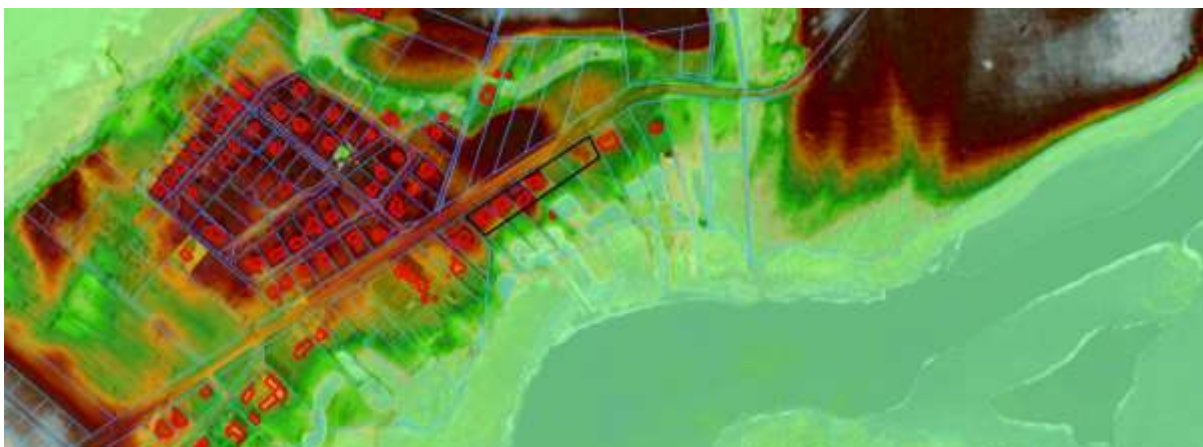
Ryc. 16. Hipsometria.
